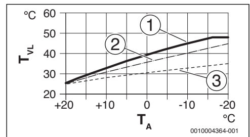
Fig. 11 Impostazione della curva termocaratteristica per impianto di riscaldamento a pannelli radianti Pendenza a salire tramite la temperatura di progetto T_{AL} e la temperatura esterna minima T_{A,min}
